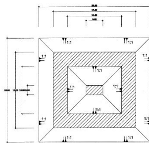
แปลนสระกับน้ำรูปสี่เหลี่ยม NO SCALE
