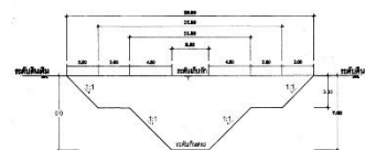
รูปตัดตามยาวสระเก็บน้ำรูปสี่เหลี่ยม ความลึก 7.00 เมตร
