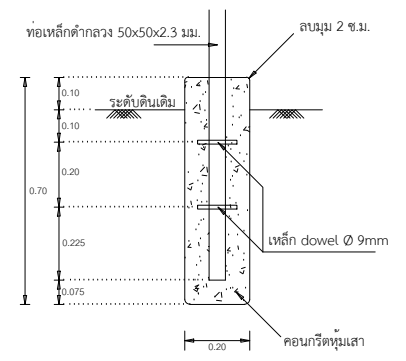
แบบขยายคอนกรีตหุ้มเสา
