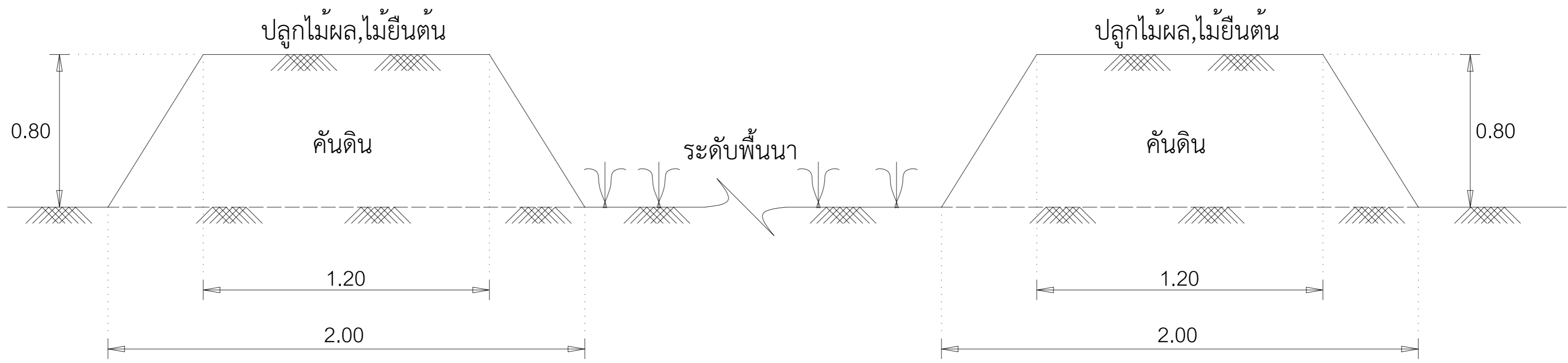
รูปตัดการปรับระดับพื้นที่นา รูปแบบที่ 1
