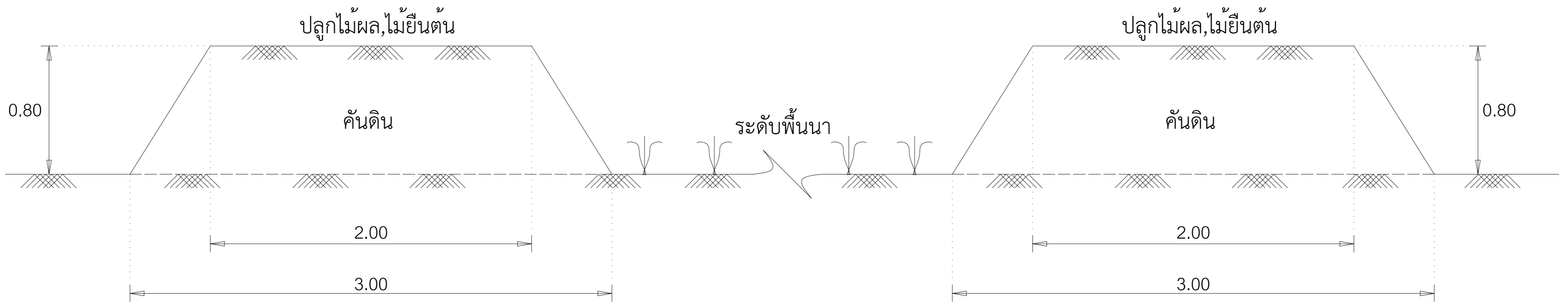
รูปตัดการปรับระดับพื้นที่นา รูปแบบที่ 2
