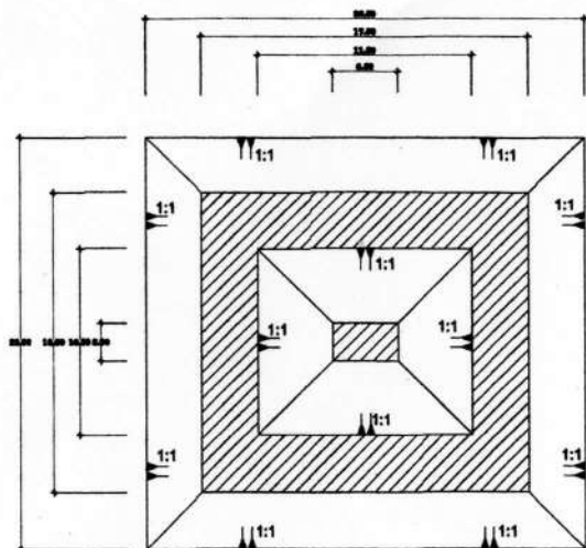
แปลนสระเก็บน้ำรูปสี่เหลี่ยม NO SCALE
