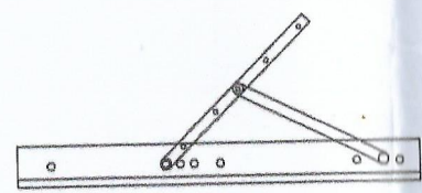
แบบขยายบานพับเหล็ก 16 นิ้ว
