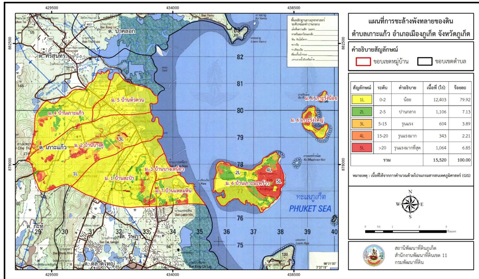
รูปที่ 7-1 การชะล้างพังทลายของดินในเขตการใช้ที่ดิน ตำบลเกาะแก้ว อำเภอเมืองภูเก็ต จังหวัดภูเก็ต
