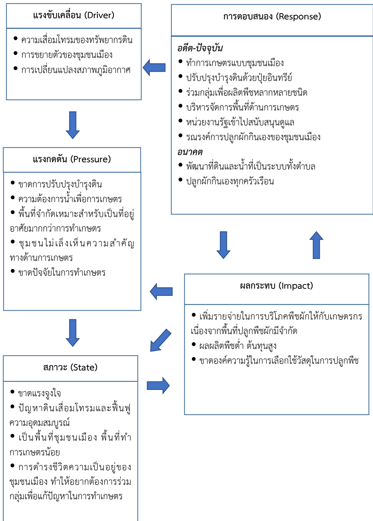
รูปที่ 4-1 การวิเคราะห์สถานการณ์โดยระบบ DPSIR ของตำบลเกาะแก้ว อำเภอเมืองภูเก็ต จังหวัดภูเก็ต
