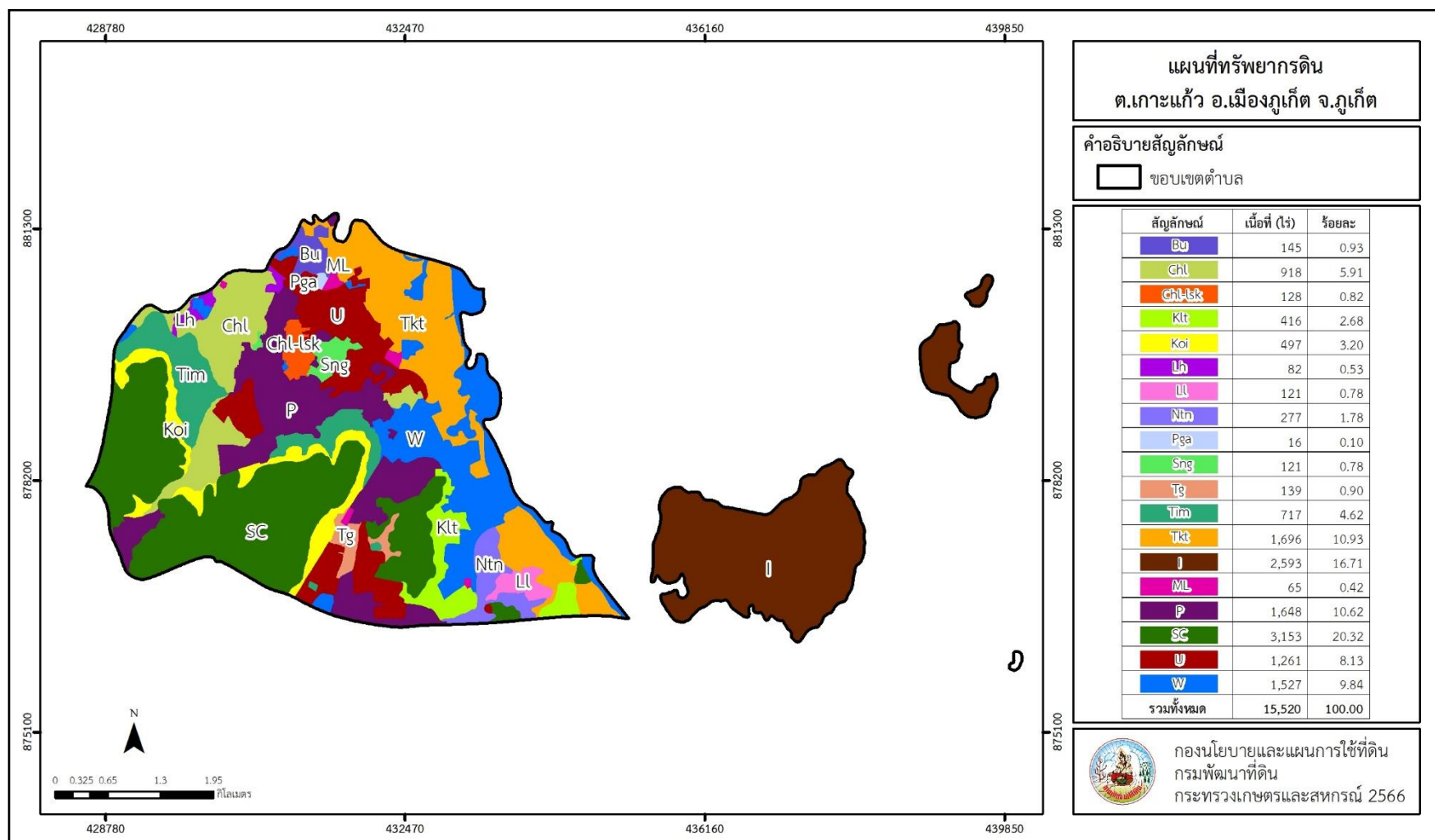
รูปที่ 3-1 ทรัพยากรดิน ตำบลเกาะแก้ว อำเภอเมืองภูเก็ต จังหวัดภูเก็ต
