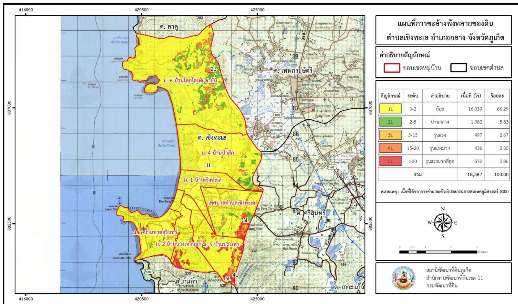
รูปที่ 7-1 การชะล้างพังทลายของดินในเขตการใช้ที่ดินตำบลเชิงทะเล อำเภอลาง จังหวัดภูเก็ต
