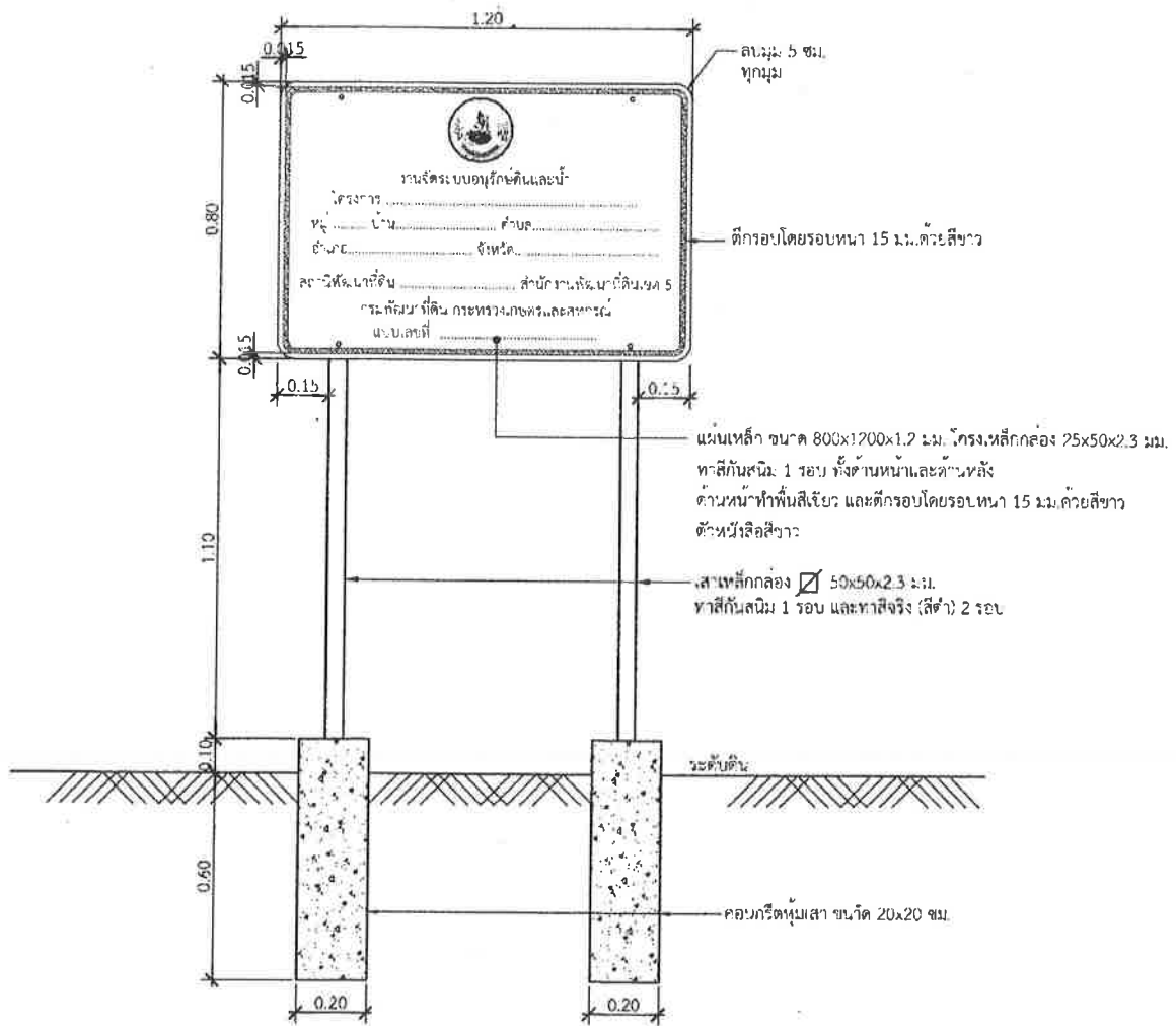
ด้านหน้า แบบป้ายโครงการ มาตรฐาน : 20
