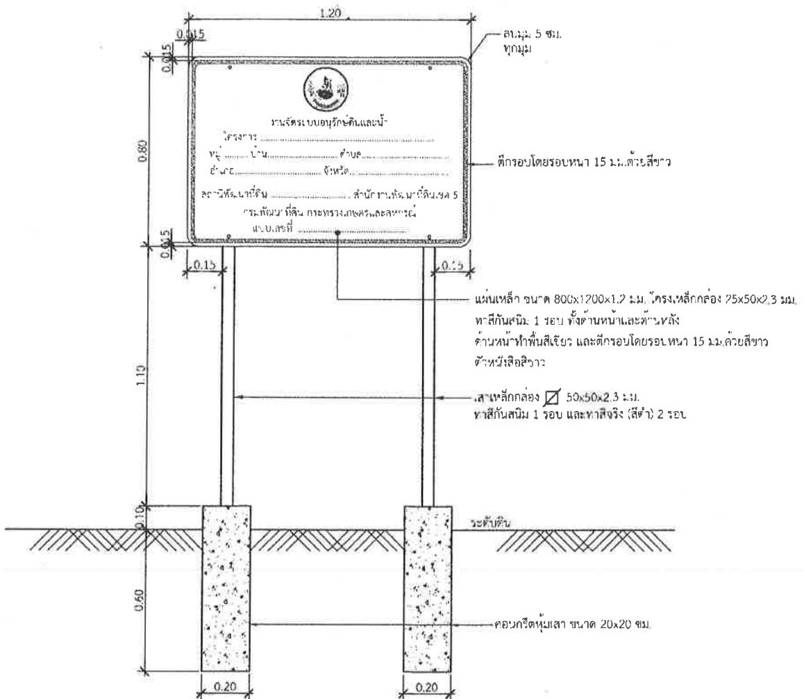
ด้านหน้า แบบป้ายโครงการ มาตราส่วน 1 : 20
