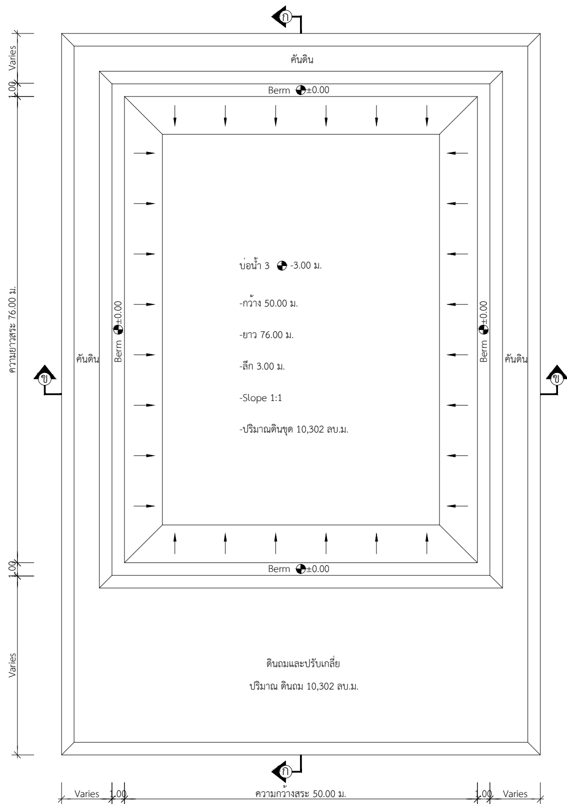
แปลนการขุดบ่อน้ำ 3
