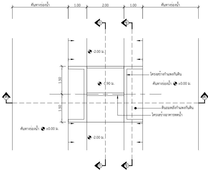
แปลนอาคารชะลอน้ำ ร่อนน้ำ 4 เมตร
