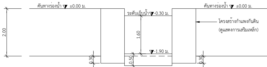
แสดงรูปทรงอาคารชะลอน้ำ
