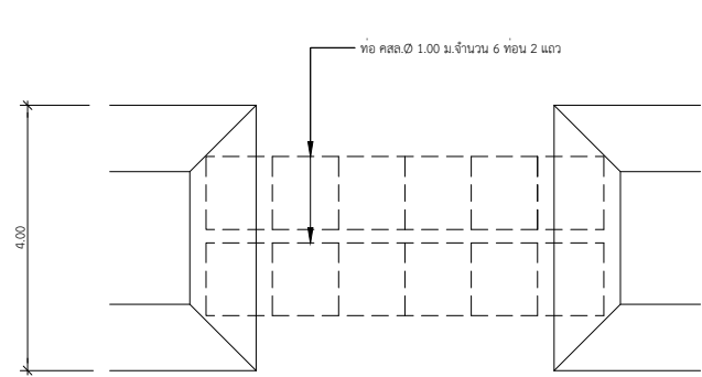
แปลนทางข้ามแบบทอลอด มาตรฐาน 1:75
