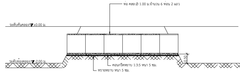
แสดงรูปตัดทางข้ามแบบทอลอด มาตรฐาน 1:75
