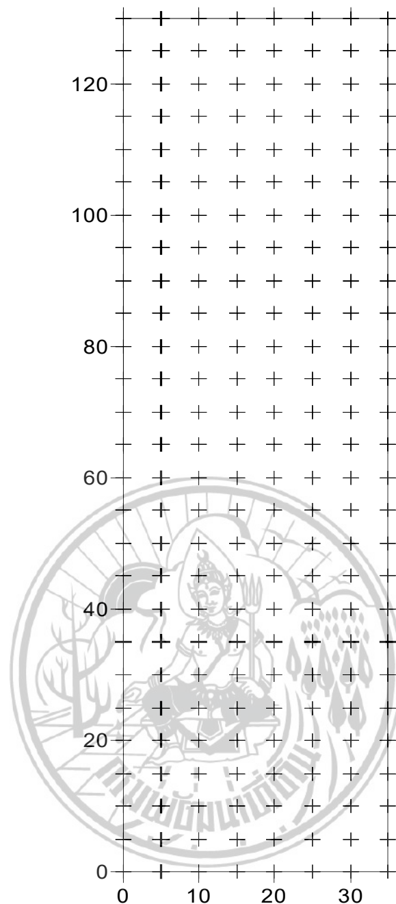
ภาพที่ 2 จุดพิกัดระยะห่าง 5 เมตร สำหรับวัดค่า EC_e ด้วยเครื่อง EM38 แปลงที่อำเภอกษัตริย์
